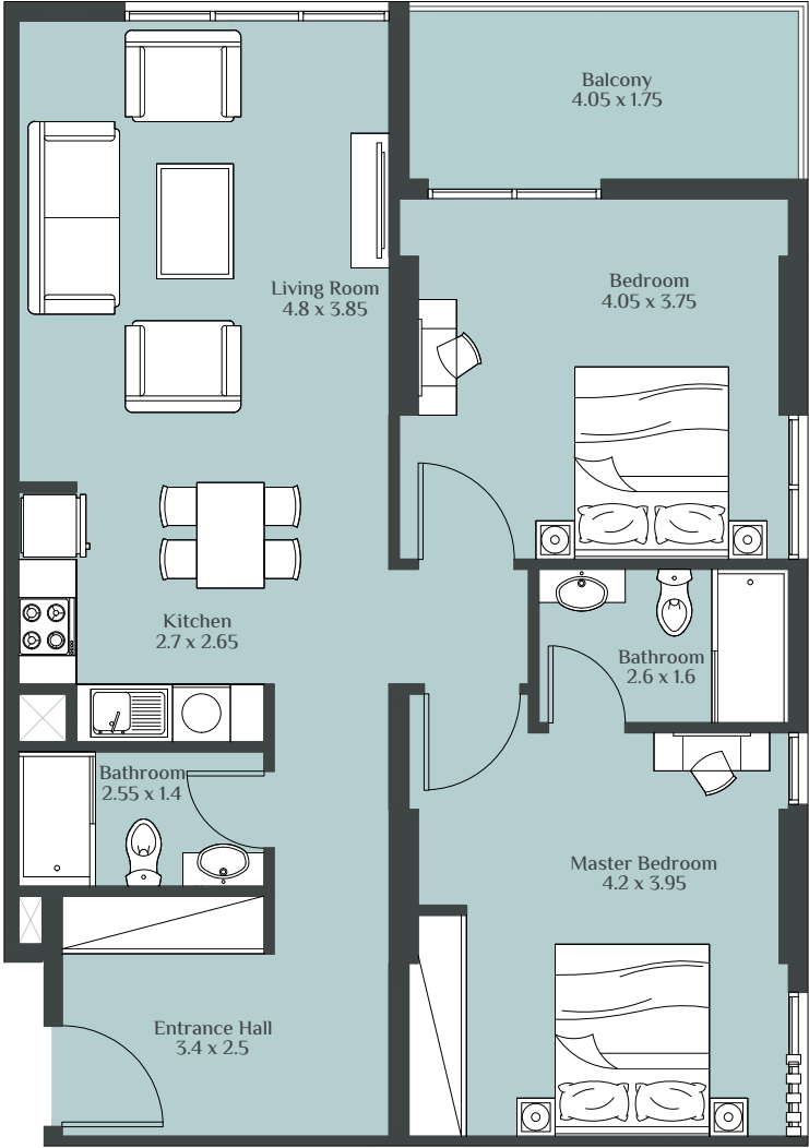
2 BEDROOM TYPE - D
